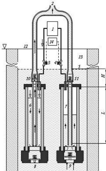
Figura 1: Esquema de armado y funcionamiento de la bomba neumática en paralelo. (1) fuente de aire comprimido; (2) salida de agua; (3) electroválvula ev1; (4) electroválvula ev2; (5) nivel de agua; (6) cámara c1; (7) cámara c2; (8) válvula de retención tr1-1; (9) válvula de retención tr1-2; (10) válvula de retención tr2-1; (11) válvula de retención tr2-2; (12) nivel del suelo; (13) perforación; (14) control automático (ctlp) de la electroválvula ab
